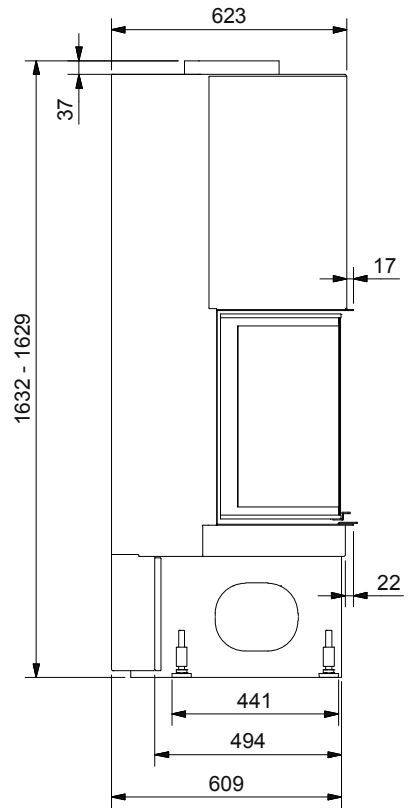
Seitenansicht / Vue de coté Vista laterale / Side view
