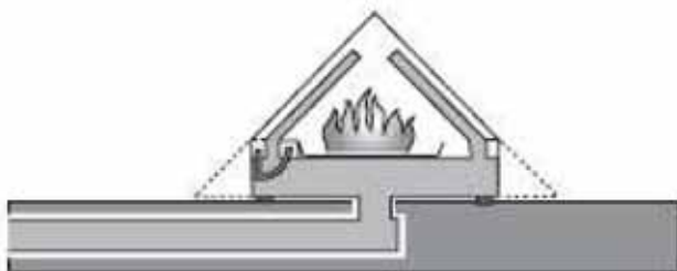
Implantació amb connexió dins del forjat
