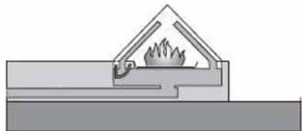
Implantació amb connexió dissimulada amb un sòcol
